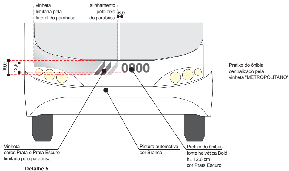
Detalhe 5
