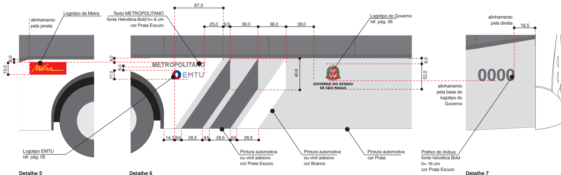
Detalhe 5
