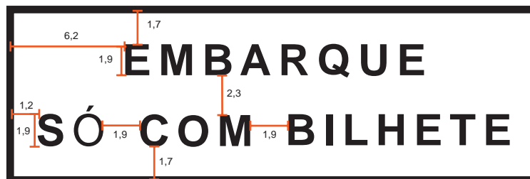
Adesivo porta dianteira
