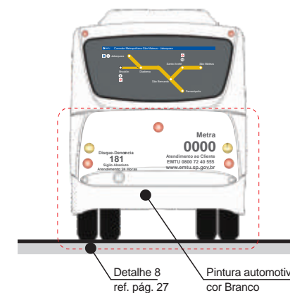
Vista traseira
