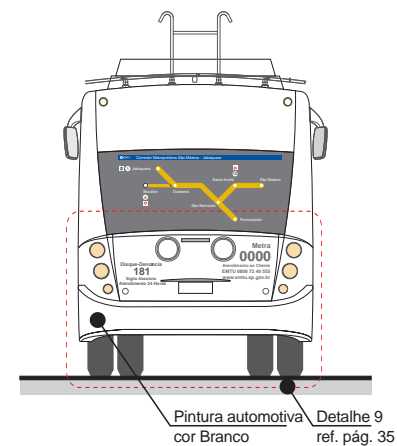
Vista traseira
