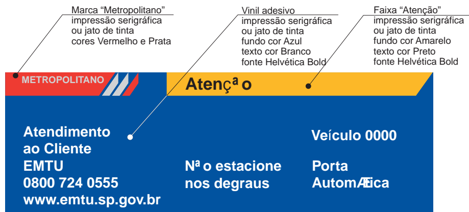
Tampa da Caixa das Portas sem o Disque-Denúncia
