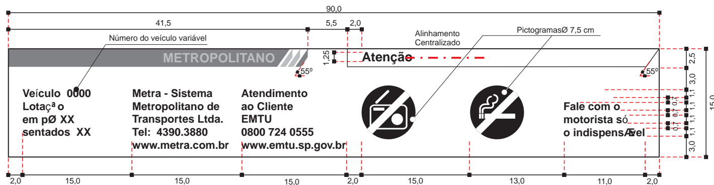
Tampa da Caixa do Letreiro
