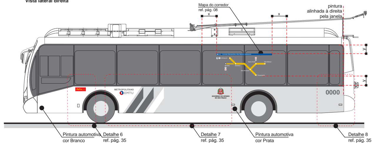
Vista lateral esquerda
